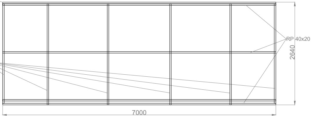
rzut przyziemia
