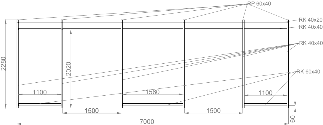
RK 40x40
