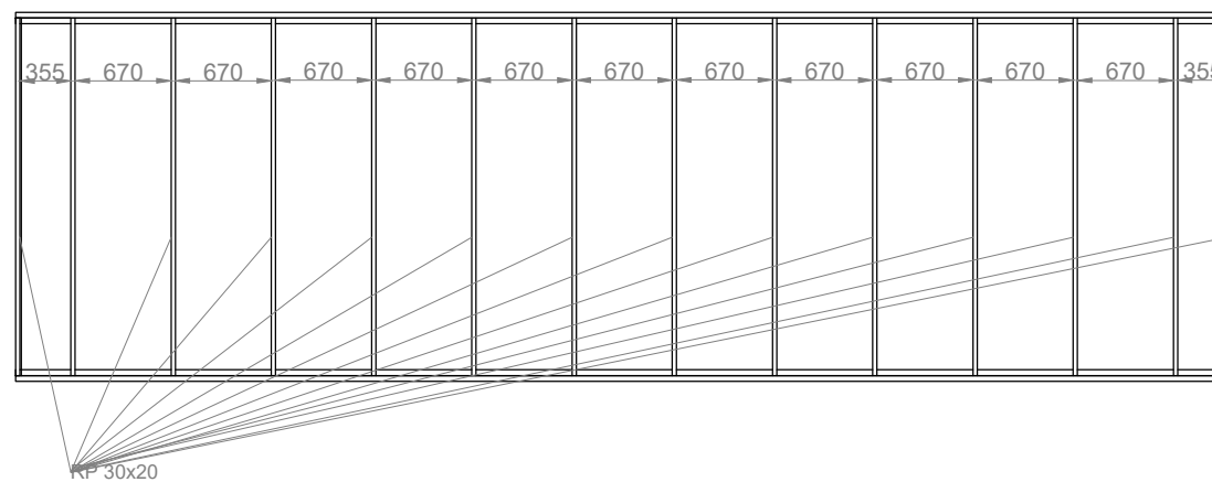
rzut dachu
