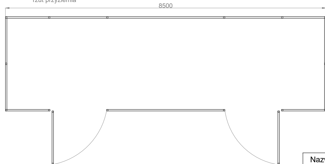
rzut przyziemia
