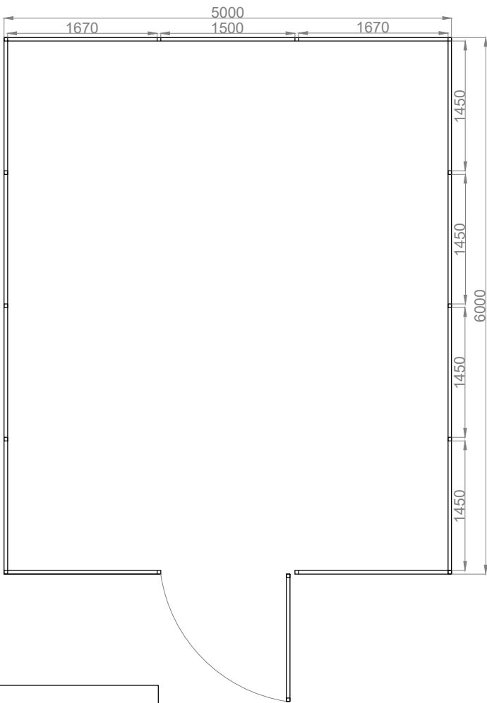
rzut przyziemia
