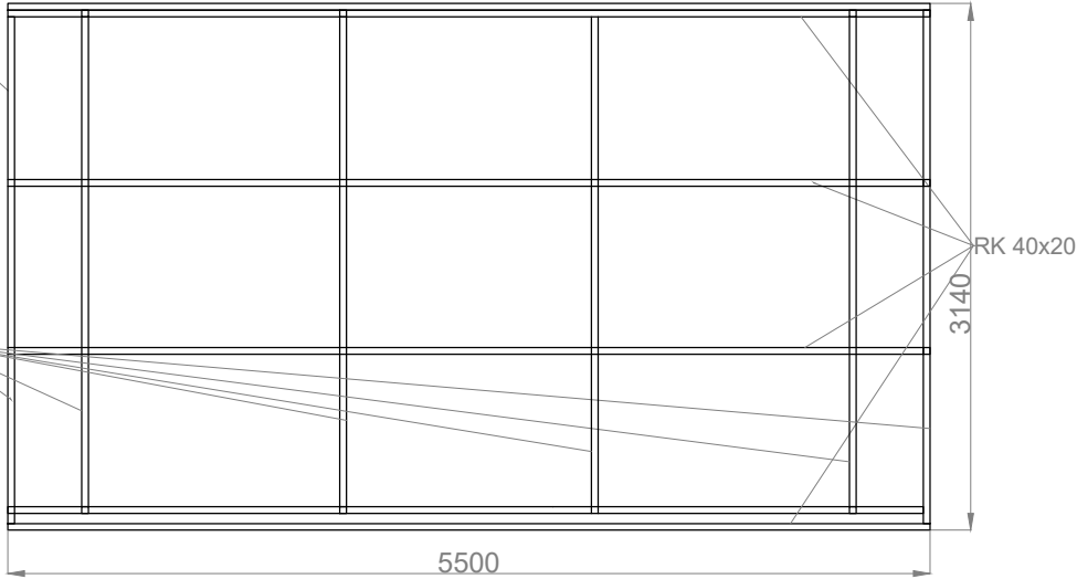
rzut przyziemia
