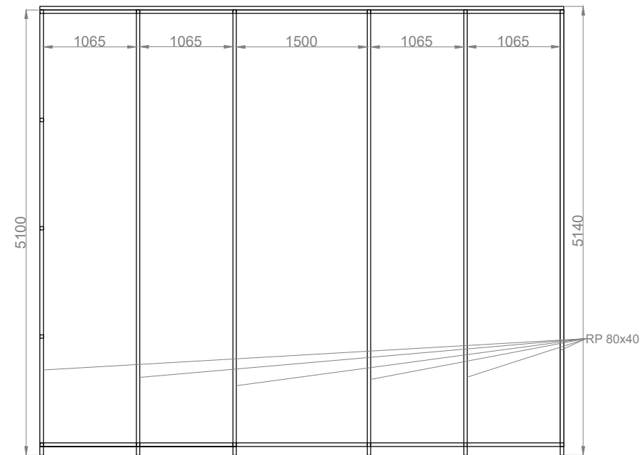
rzut dachu
