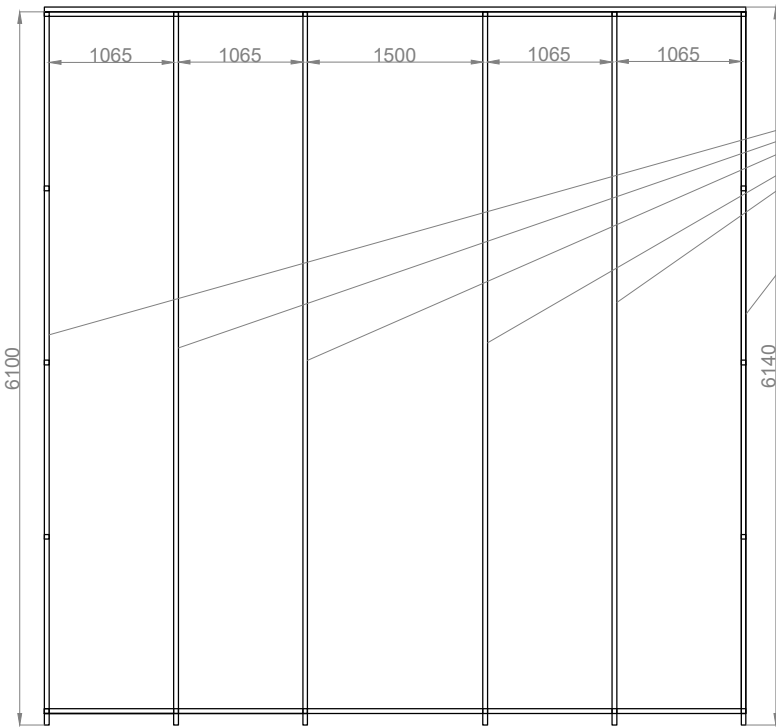
rzut dachu
