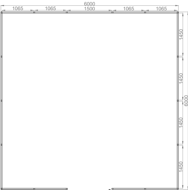
rzut przyziemia
