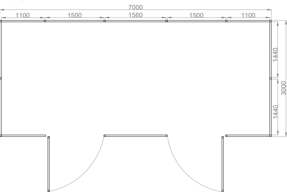
rzut przyziemia
