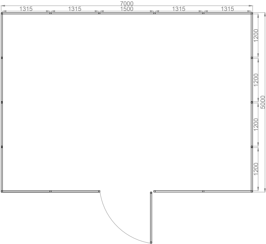
rzut przyziemia
