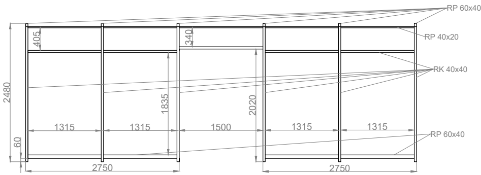
rzut dachu
