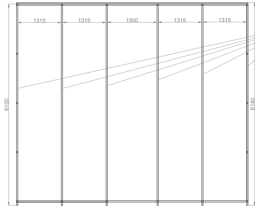
rzut dachu
