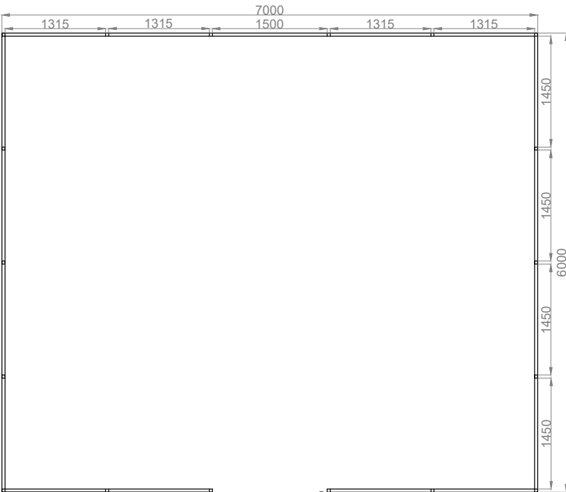
rzut przyziemia
