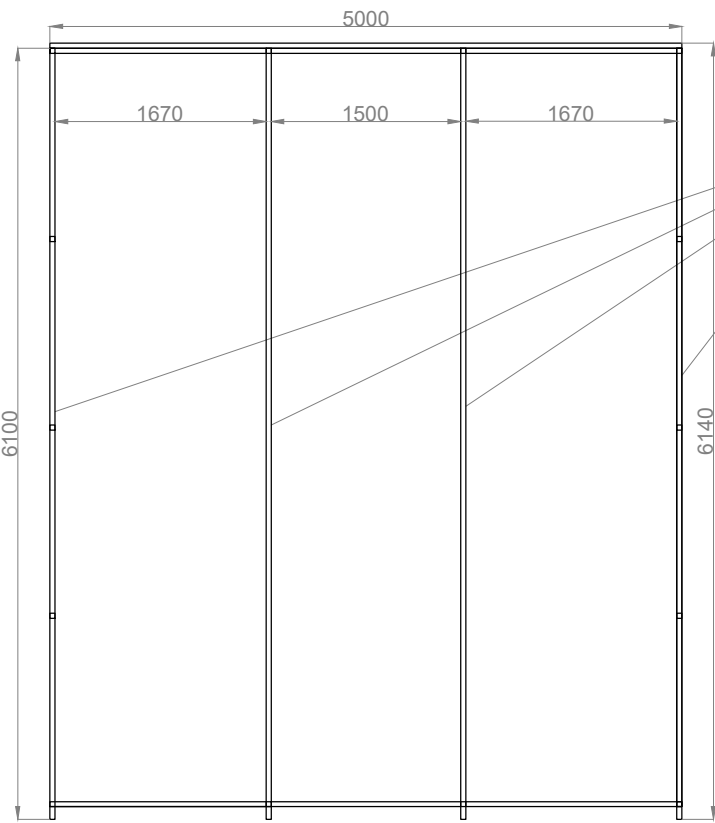
rzut dachu
