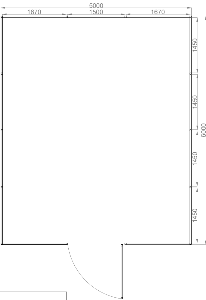
rzut przyziemia
