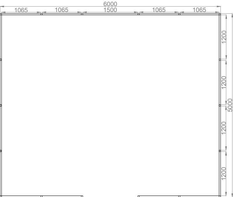
rzut przyziemia
