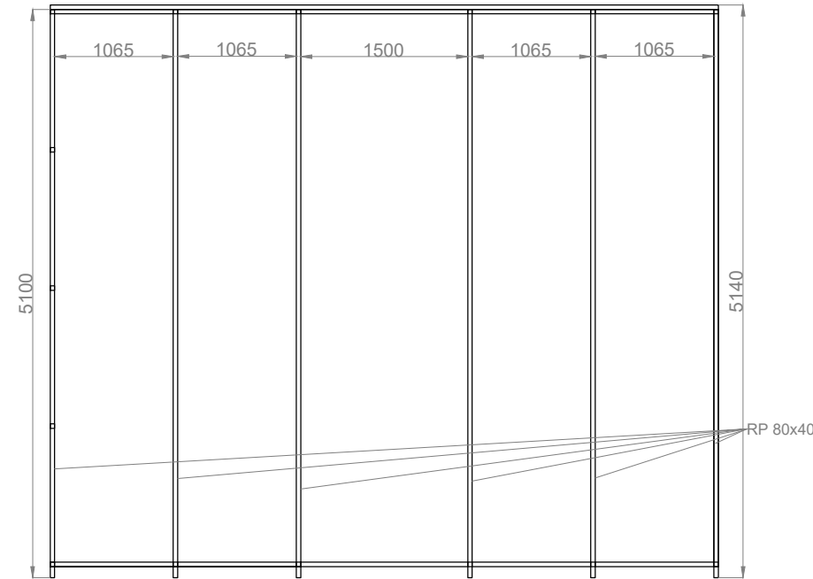
rzut dachu
