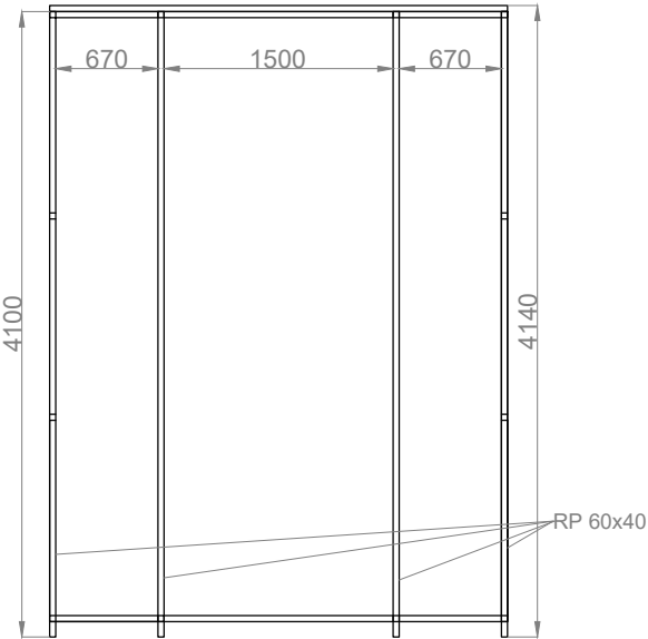
rzut dachu
