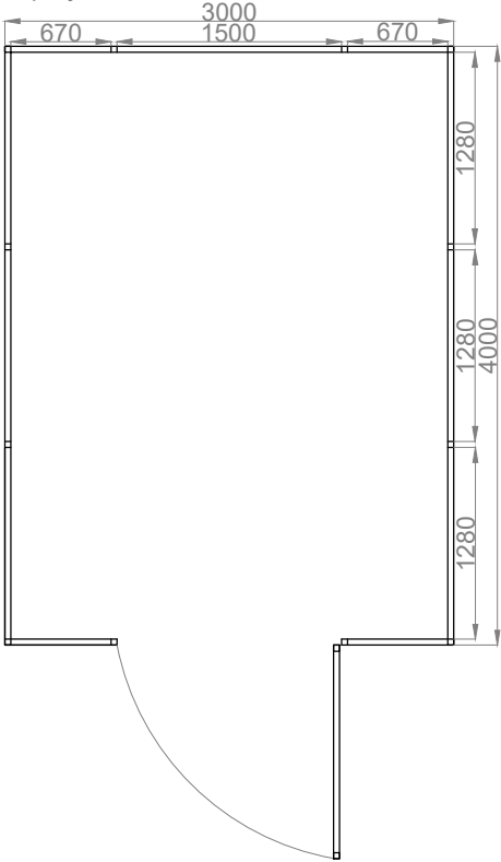
rzut przyziemia
