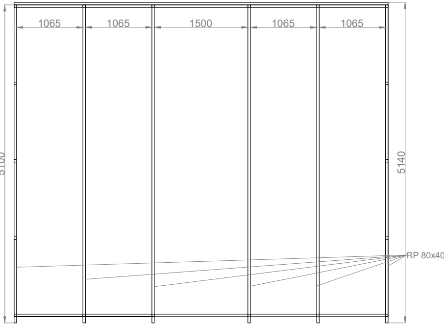
rzut dachu
