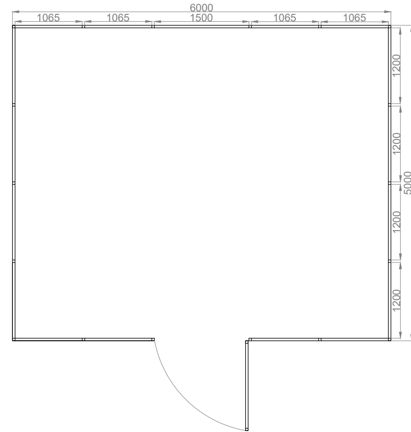
rzut przyziemia
