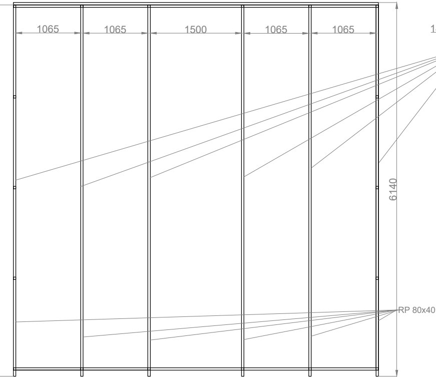
rzut dachu
