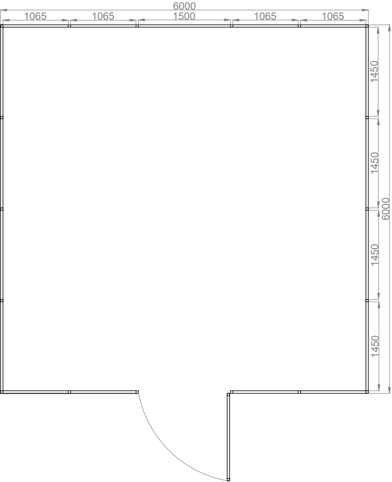
rzut przyziemia
