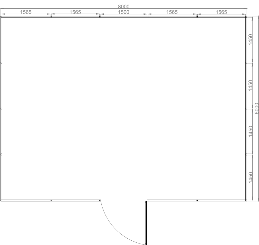
rzut przyziemia
