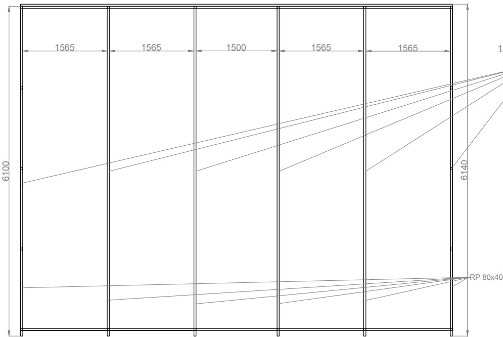
rzut dachu
