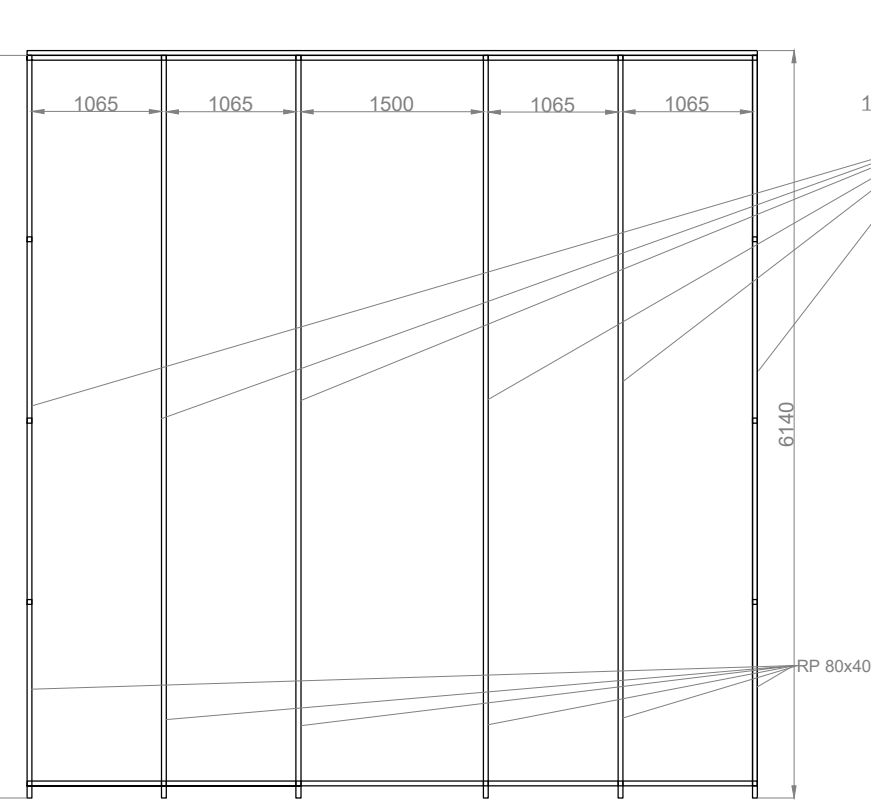
rzut dachu
