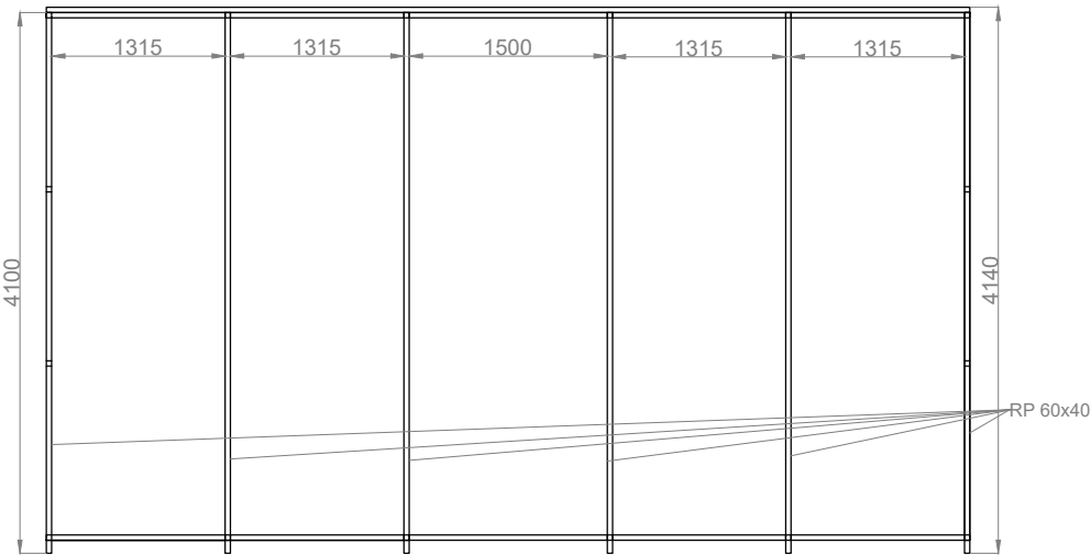
rzut dachu
