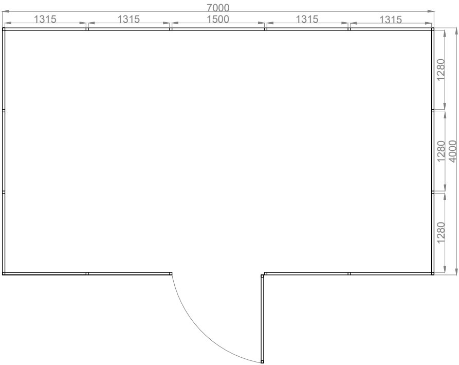
rzut przyziemia
