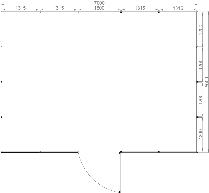
rzut przyziemia
