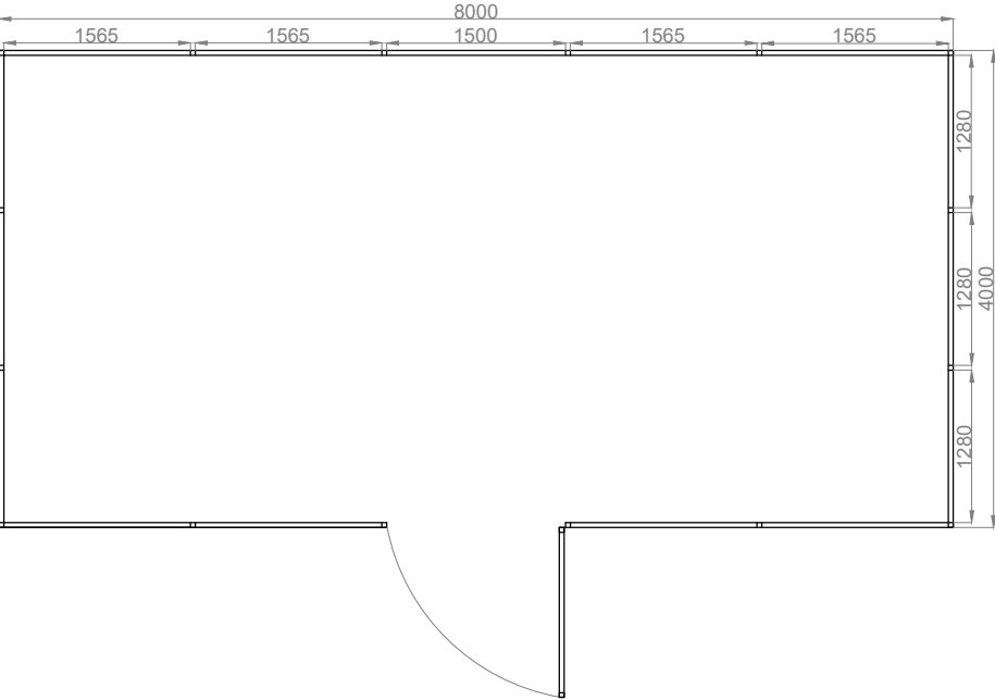
rzut przyziemia
