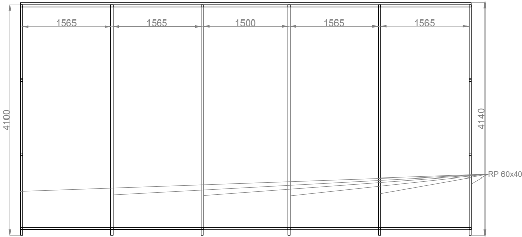
rzut dachu
