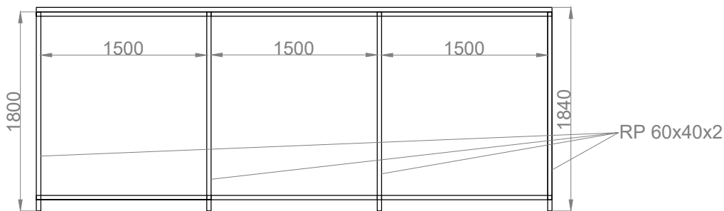
rzut dachu
