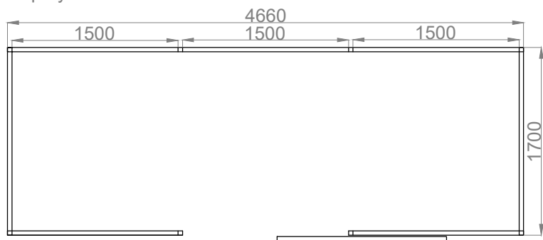
rzut przyziemia
