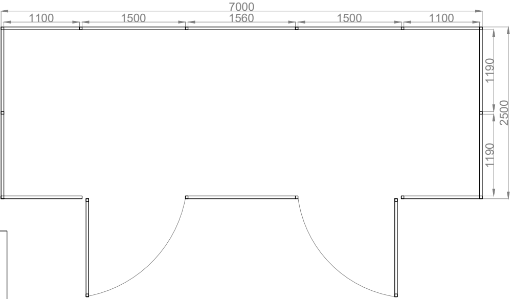
rzut przyziemia
