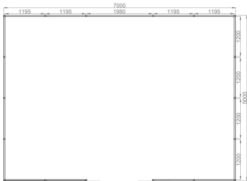
rzut przyziemia
