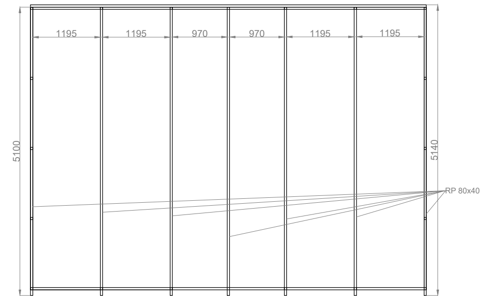
rzut dachu
